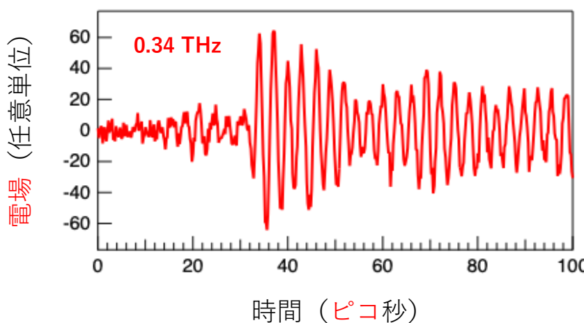
図1 半導体テラヘルツ発振器から放射されたテラヘルツ電磁波の振動電場波形。 数ピコ秒（1ピコ秒は0.000000000001秒）周期の超高速振動波形が変化の様子を捉えた。
